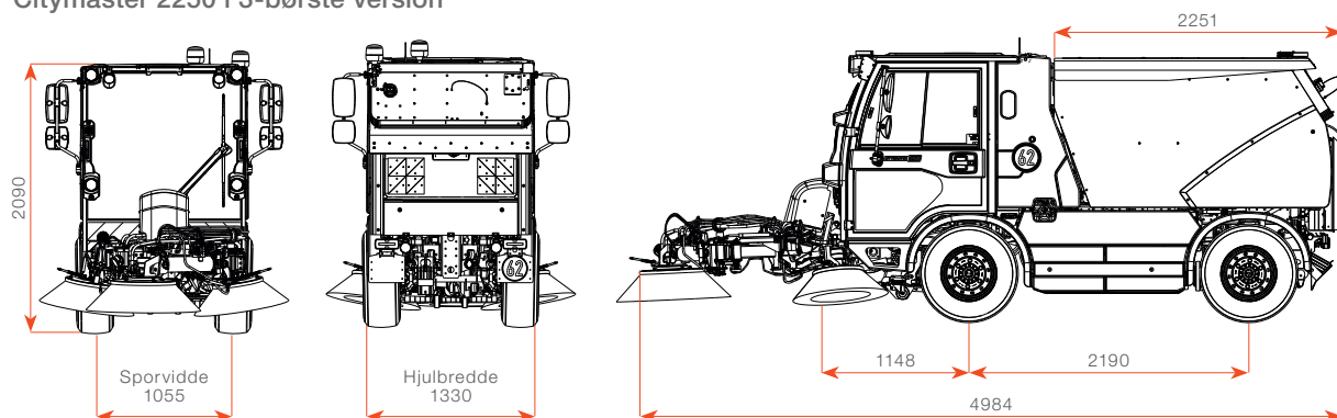
Citymaster 2250 i 3-børste version
