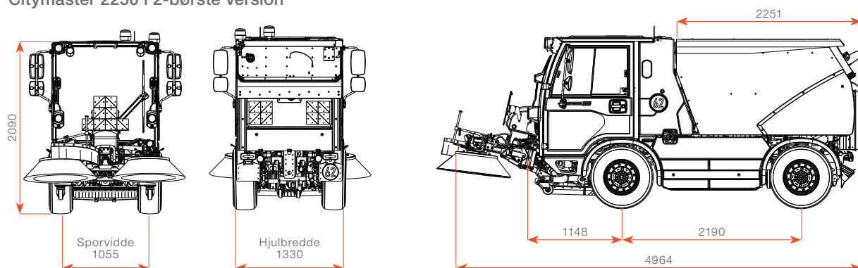
Citymaster 2250 i 2-børste version
